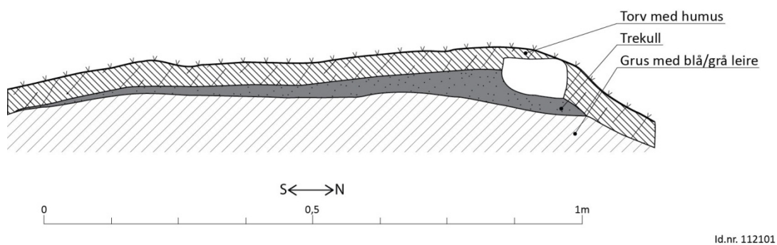
Figur 20 Id.nr. 112101 profiltegnig
