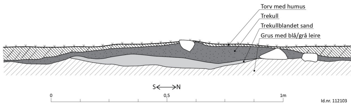
Figur 24 Id.nr. 112103 profiltegnig
